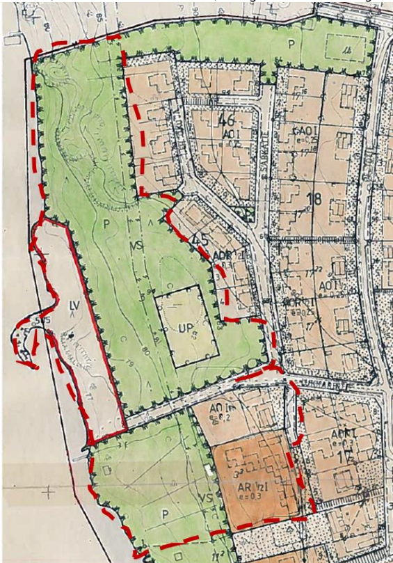
Kuva 5: Ote ajantasa-asetmakaavasta. Muutosalue osoitettu punaisella katkoviivalla.
